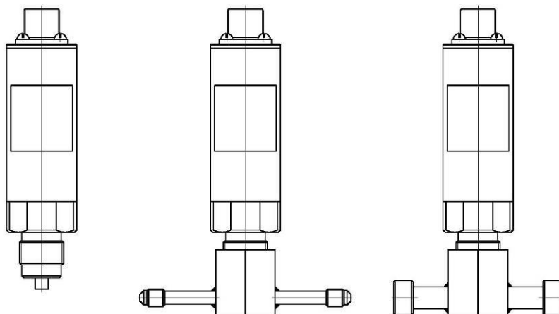
Рисунок 3.16 Измерительные преобразователи давления ИПД-02, ИПД-02-M8, ИПД-02-M16 (по порядку слева направо)
