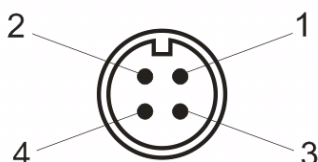
Рисунок 3.5 Разъем подключения преобразователей давления
