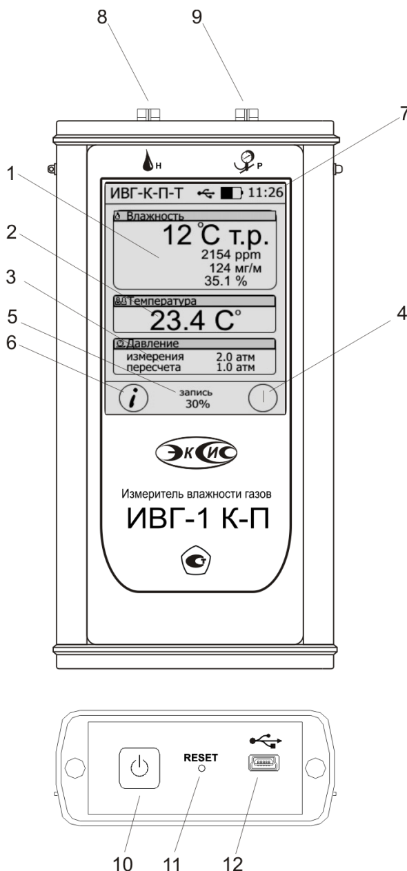
Рисунок 3.1 Вид лицевой панели прибора
